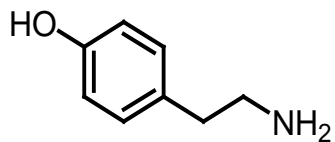
Tyramine
